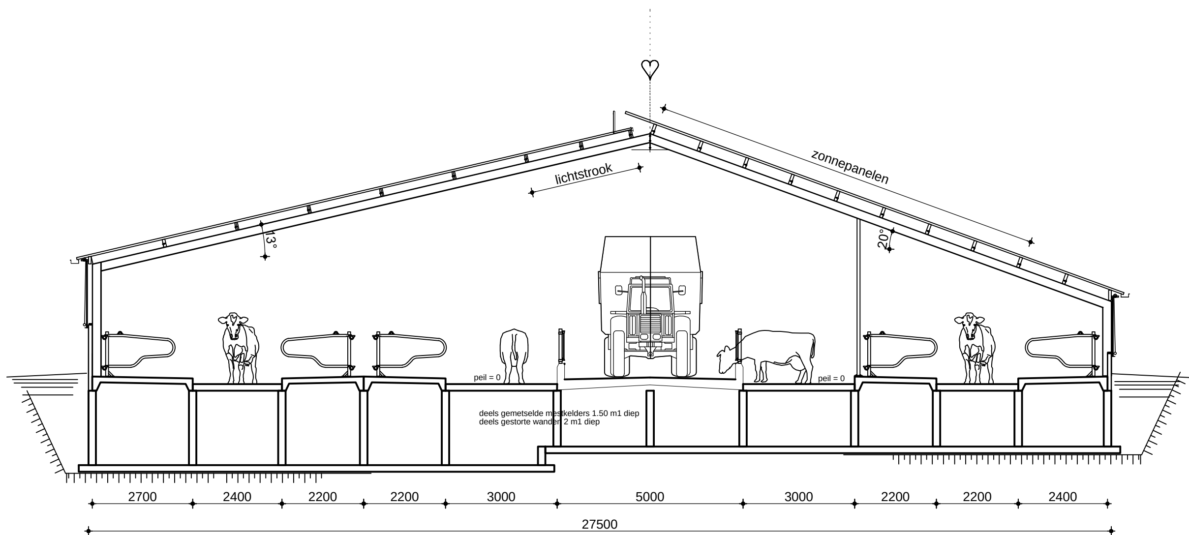
bestaande doorsnede
