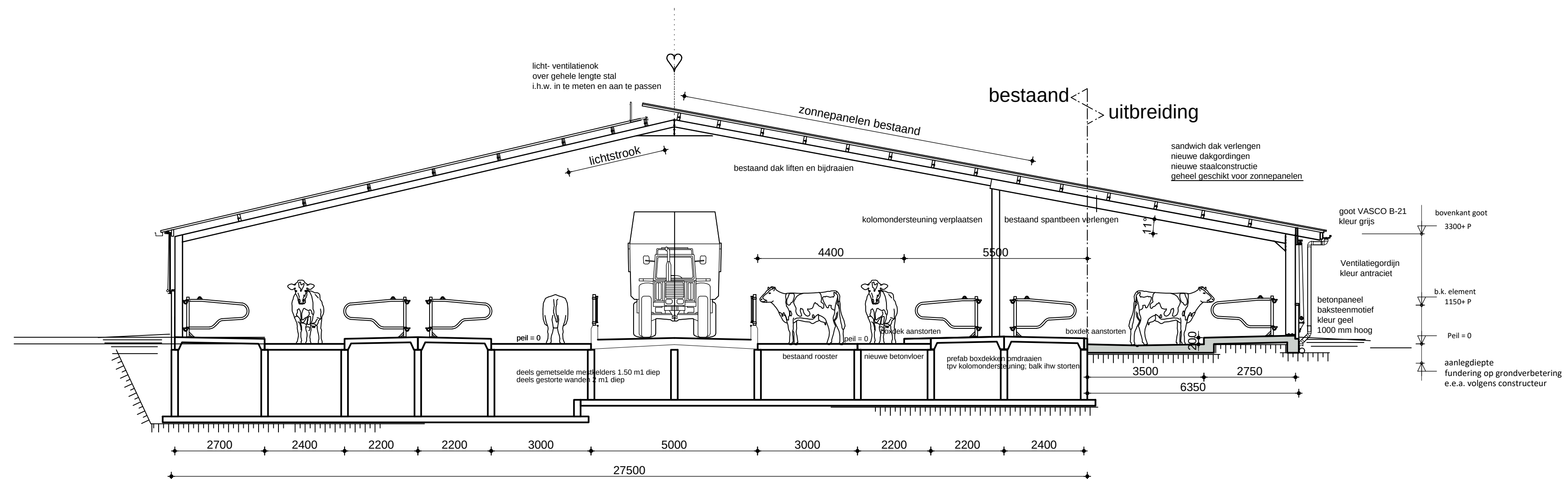
nieuwe doorsnede (uitbreiding bestaande zijgevel)
