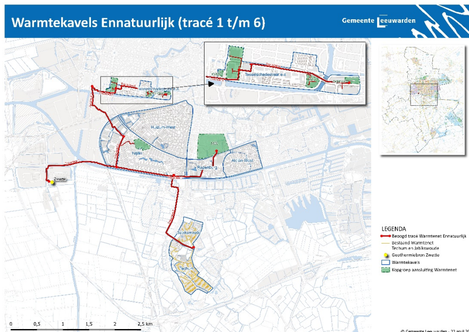
Figuur 1: Beoogd hoofdtracé warmtenet Ennatuurlijk en beoogde warmtekavels
